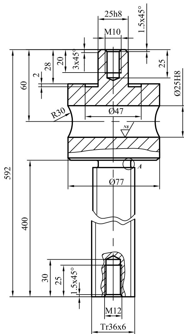
DETALJ A 2:1
